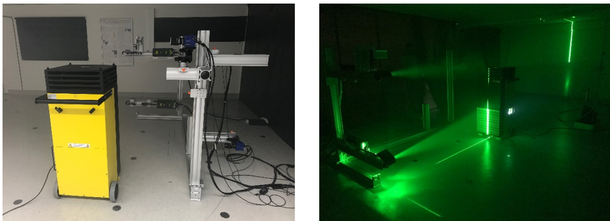
Abbildung 3: Experimenteller Aufbau mit Raumlufthereiniger, zwei Doppelpulslasern und 4 sCMOS Kameras (links) und Aufnahme während der Messung mit PIV (rechts)
